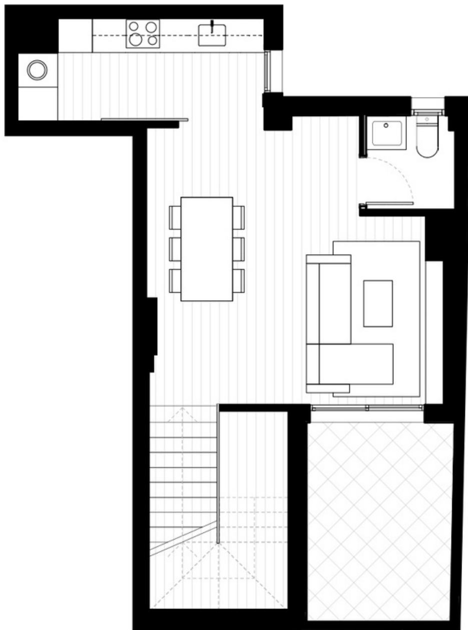
Planta Dúplex
