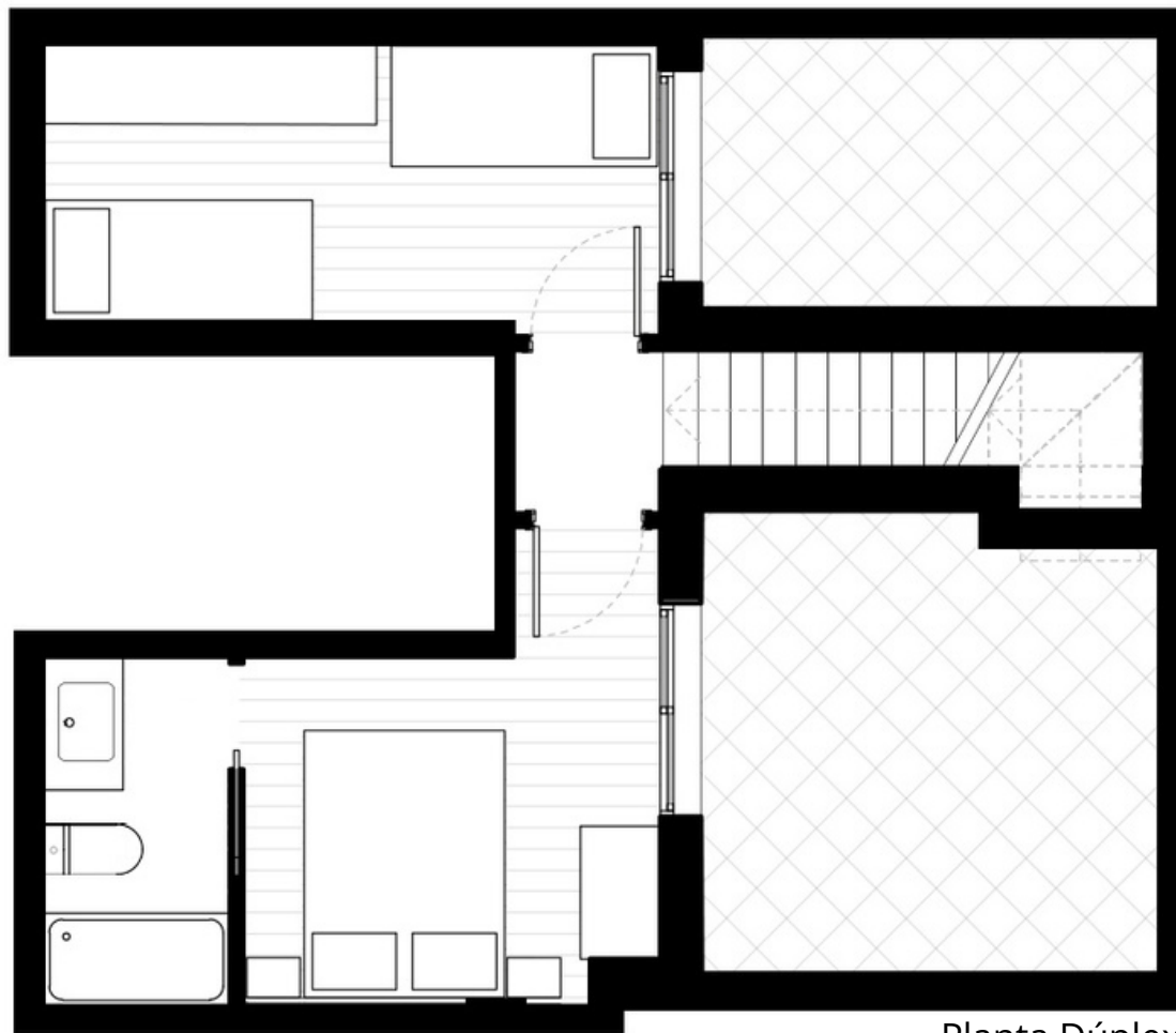
Planta Dúplex
