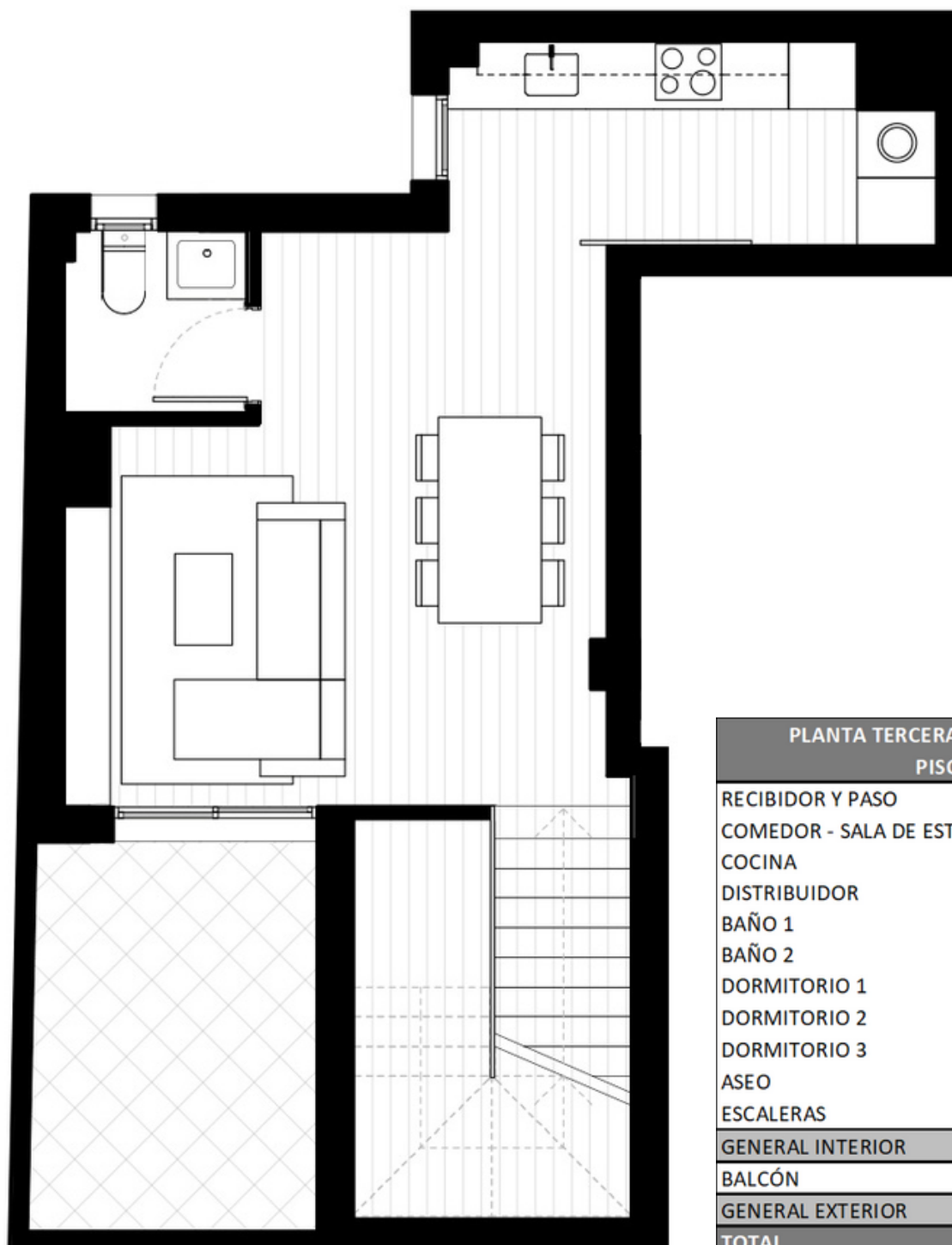
Planta Dúplex
