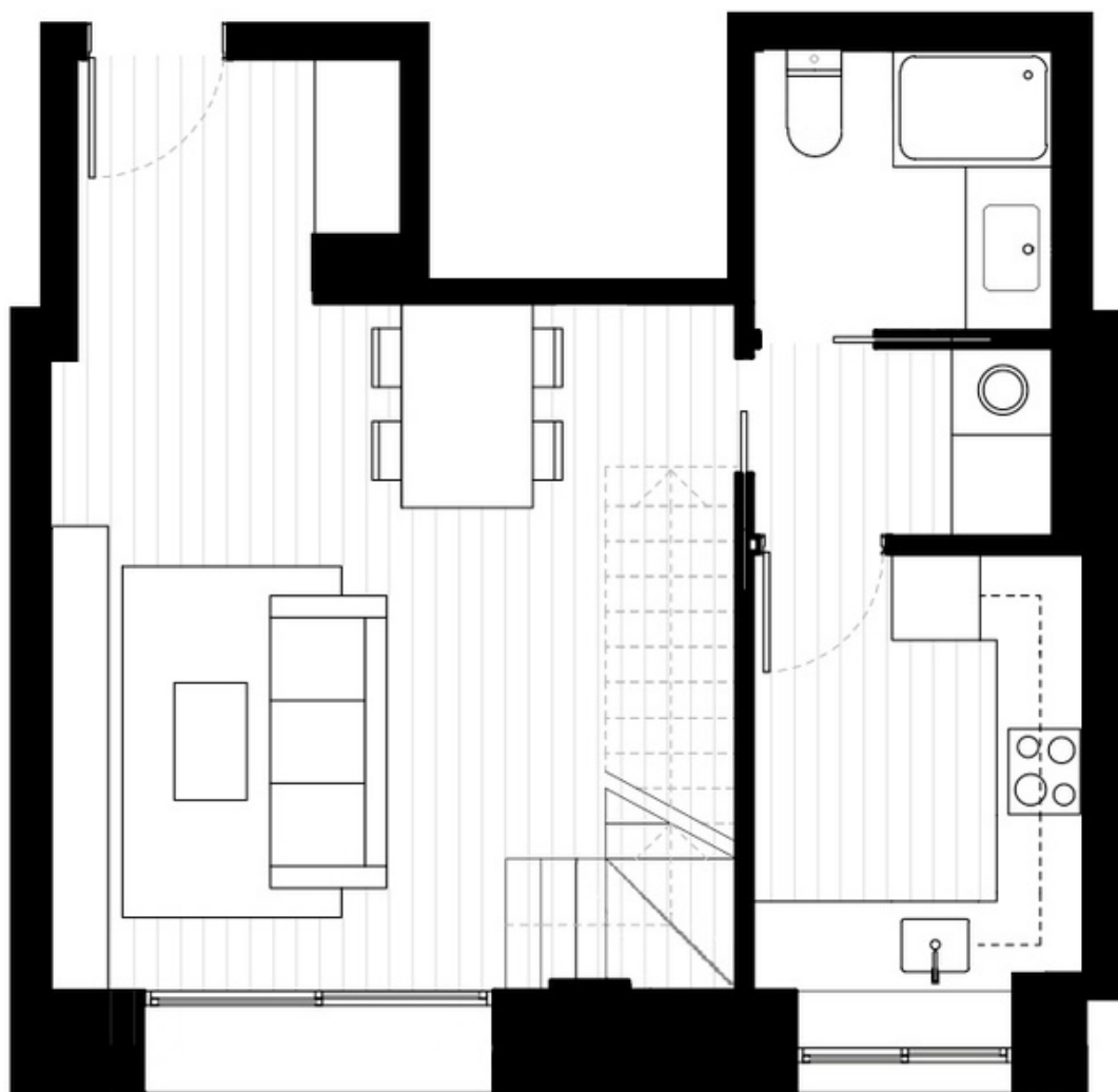
Planta 3ª
