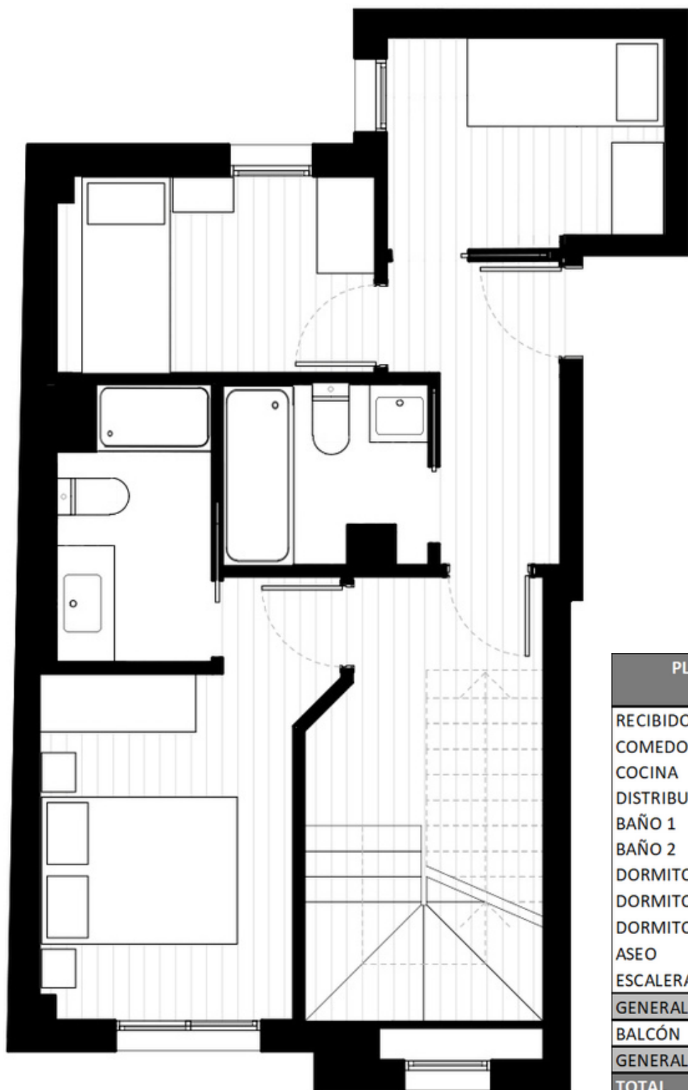
Planta 3ª
